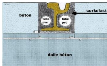
Schéma rail à gorge avec corkelast
