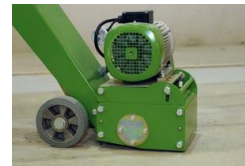
Scarificateur
